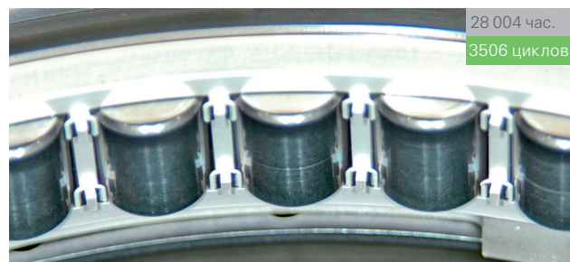
CF6-80C2, подшипник № 6 в маслоотстойнике
