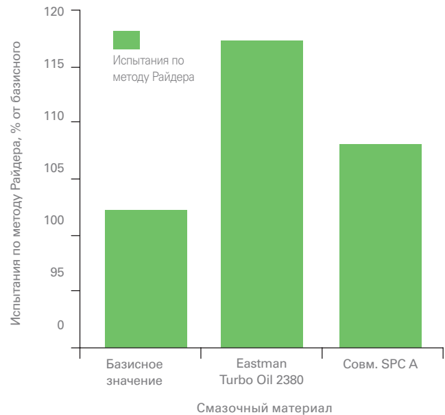
Испытания по методу Райдера
