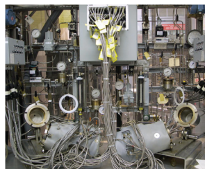
Испытательный аппарат Coker Mister
