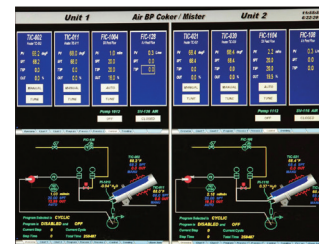
Улучшенная панель управления и мониторинга Coker Mister
