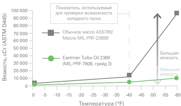
Масло Eastman Turbo Oil 2389 обеспечивает значительное преимущество при пуске при низких температурах
